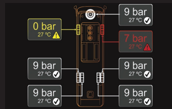
Hệ thống giám sát áp suất lốp
